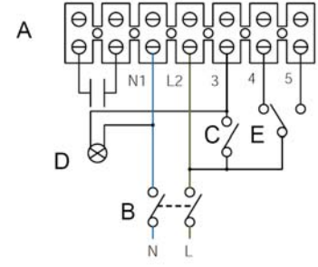
Zapojenie dvojotáčkové s časovým dobehom
