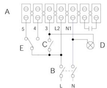
Zapojenie dvojotáčkové so svetlom a s časovým spínačom
