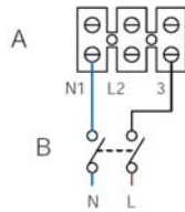
Nízke otáčky
