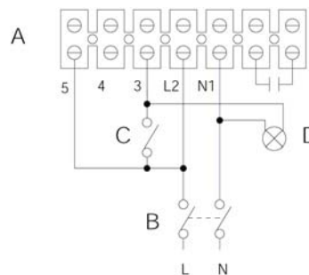
Nízke otáčky pri zapojení so svetlom
