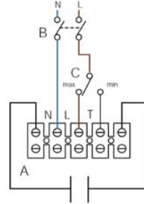
Nízke otáčky s časovým dobehom
