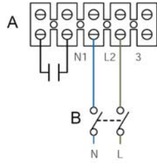
Vysoké otáčky
