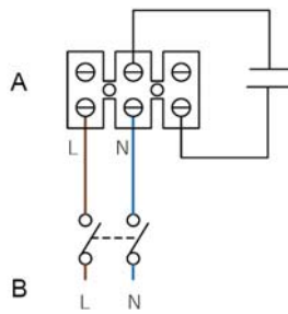
Vysoké otáčky s časovým spínačom
