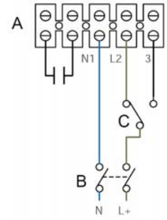
Zapojenie dvojotáčkové
