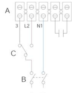
Zapojenie dvojotáčkové s časovým spínačom
