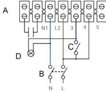
Vysoké otáčky s časovým spínačom
