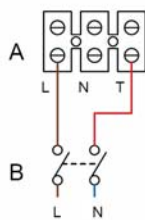
Nízke otáčky
