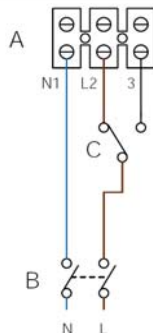
Zapojenie dvojitáčkové
