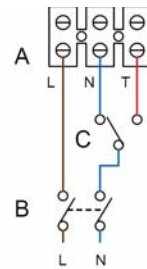
Zapojenie dvojitáčkové
