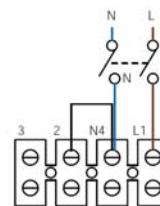
Prívod
