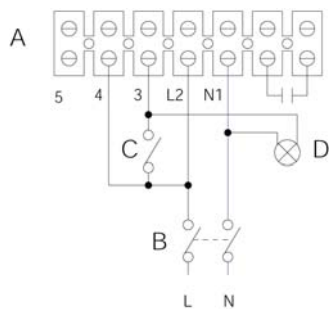
Vysoké otáčky pri zapojení so svetlom
