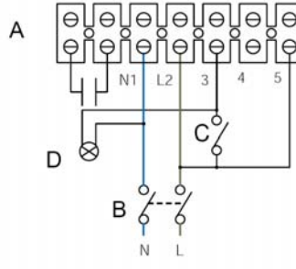
Nízke otáčky s časovým dobehom
